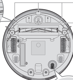
Сенсор распознавания перепадов высоты. Контакты подзарядки.
