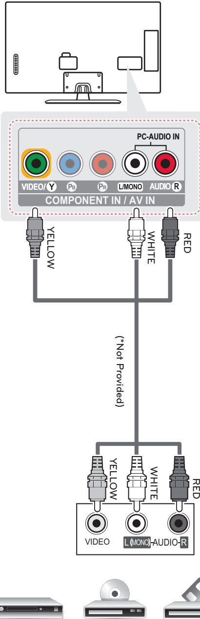
VCR / DVD / Blu-Ray / HD Cable Box
