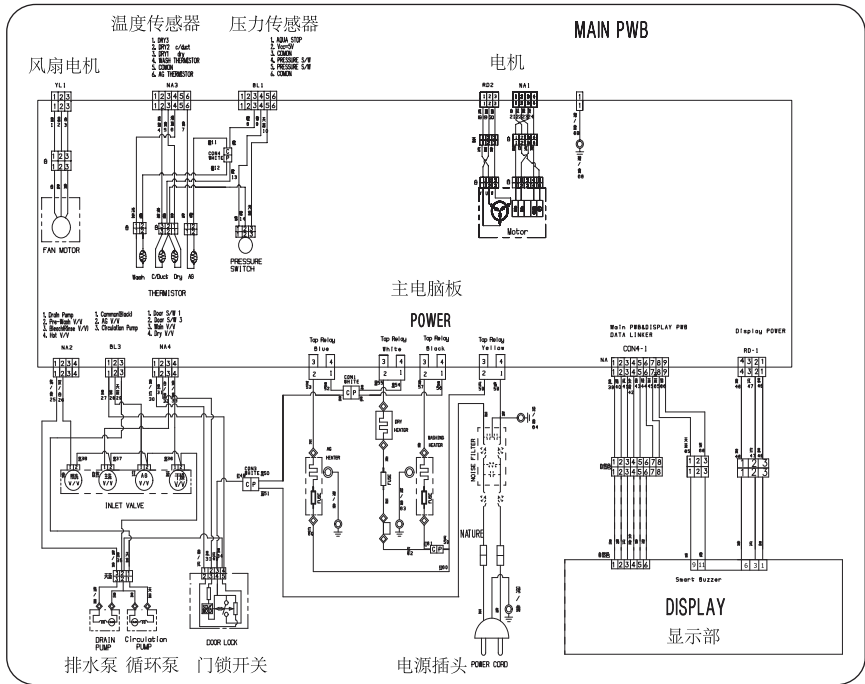
5-2 电路原理图
