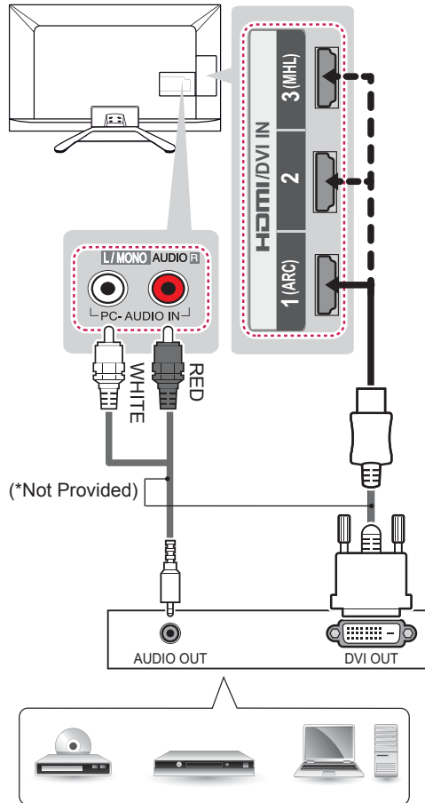
DVD/ Blu-Ray / HD Cable Box / PC
