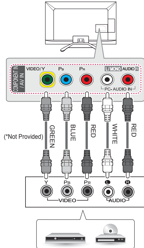
DVD/ Blu-Ray / HD Cable Box
