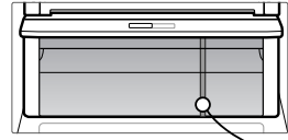
Partitioner
