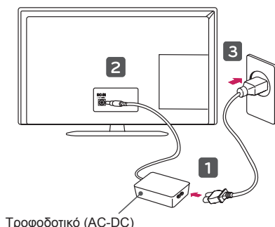
Τροφοδοτικό (AC-DC)
