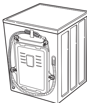
Arrière de la machine à laver
