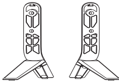
Suport Assy (Corpul suportului / Baza suportului) (Doar 70LB65**-ZA, LB67**, LB68**, LB69**, LB73**-ZA) (Consultați p. A-3)
