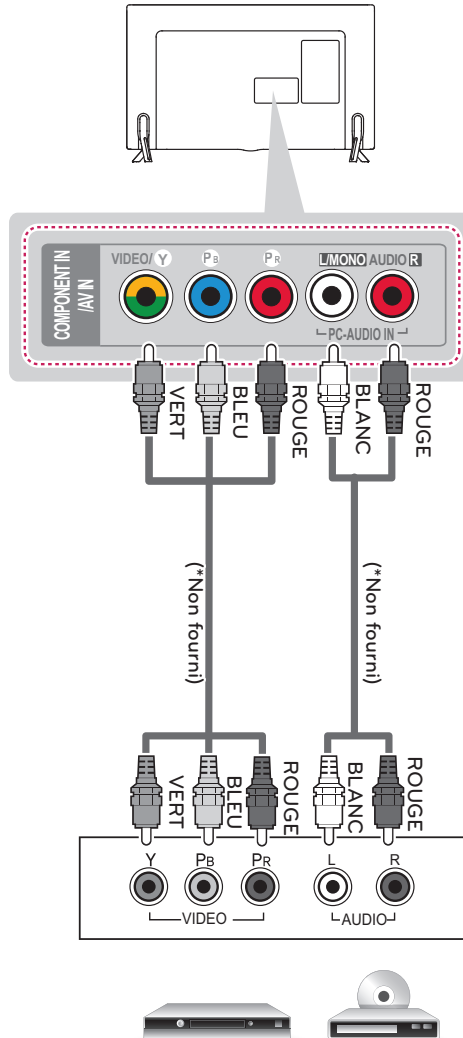
Lecteur DVD / Lecteur Blu-Ray / Câblodélecteur HD
