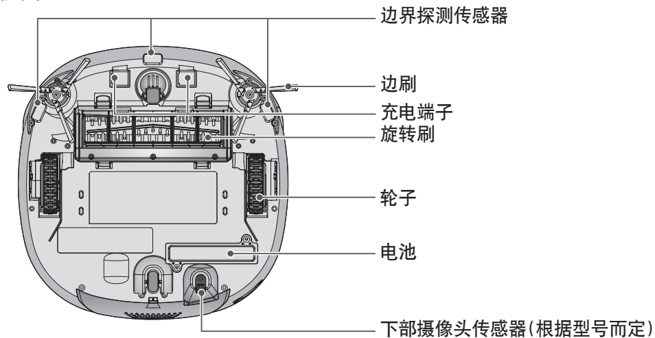
底视图
