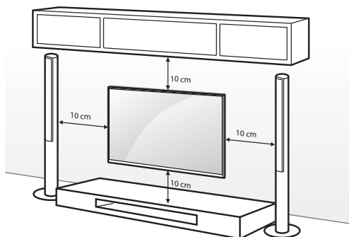
Instalação do aparelho na parede.
