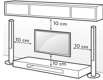
Instalação do aparelho na parede.
