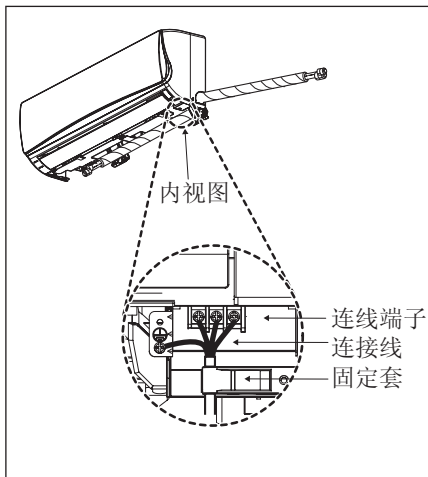
〈右方管道〉
