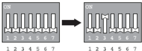
Interruptor DIP da unidade externa
