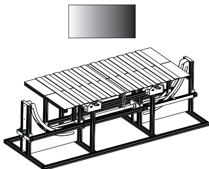
B-1 (平面夹具)
