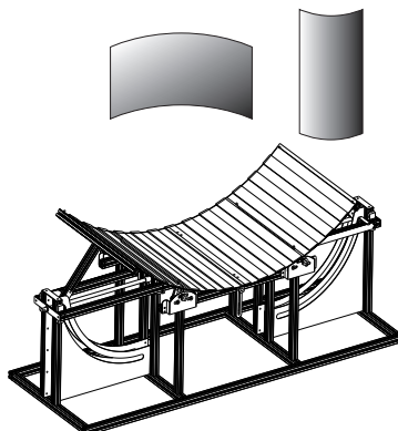
B-1 (凸面弯曲夹具)
