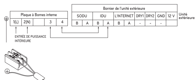
Câble blindé à deux conducteurs
