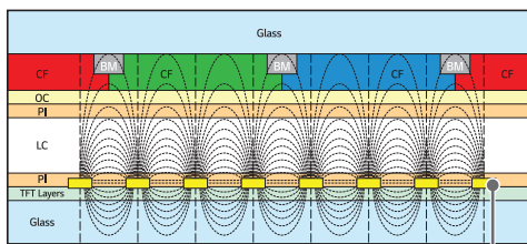
ITO 或 MoTi Pixel Layer
