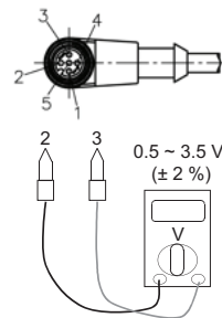
Проверете напрежението
