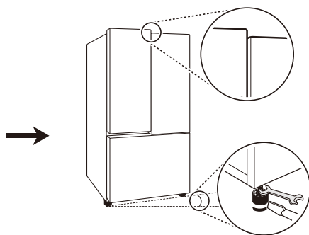
Nivellement et alignement de la porte
