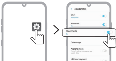
(Android 手机)
