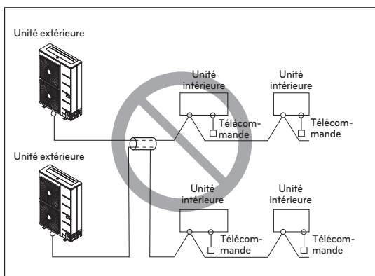
Câble multipolaire
