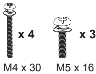
Parafuso de montagem (Apenas 42/50PM47**, 50/60PM67**, 50PM68**, 50PM97**) (Consulte a p. A-3)
