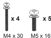
Завртки за составување (Само 60PM68**, 60PM97**) (Погледнете на стр. A-3)
