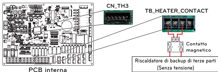
PCB interna
