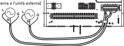
Riscaldatore di riserva 1Ø (per unità interne Split R410A serie 5, per unità interne Split R32 serie 5)
