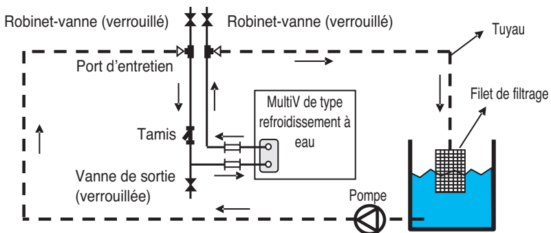
[Nettoyage de l'échangeur de chaleur radiant]
