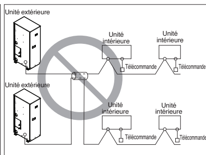
Câble multipolaire
