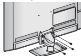
M4 X 14 (Sólo 26LE3***, 26LE5***)
