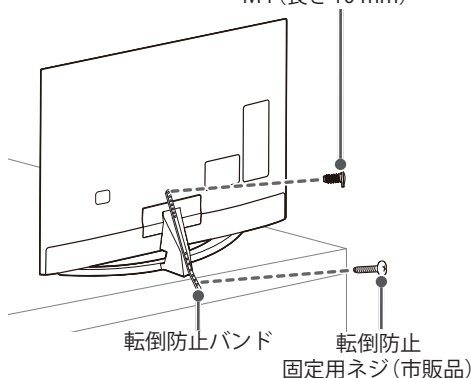
転倒防止バンド取付用ネジ M4 (長さ 10 mm)
