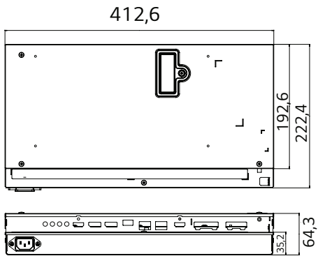
Decodificador
