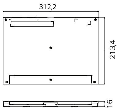
Caja T-con
