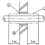
Porzione di infiltrazione alle fiamme parete di limitazione
