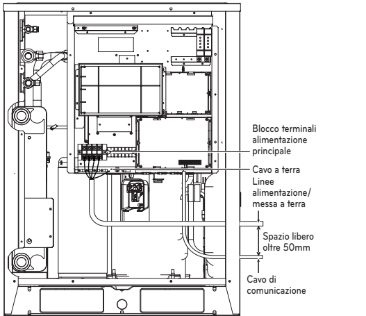
Collegamento alimentazione principale
