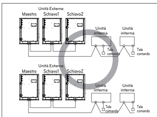
Cavo schermato a 2 conduttori
