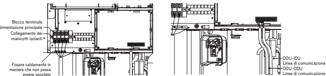
Collegamento alimentazione principale
