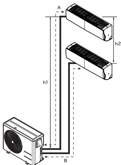
Tipo a più tubature
