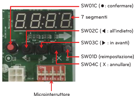
Microinterruttore
