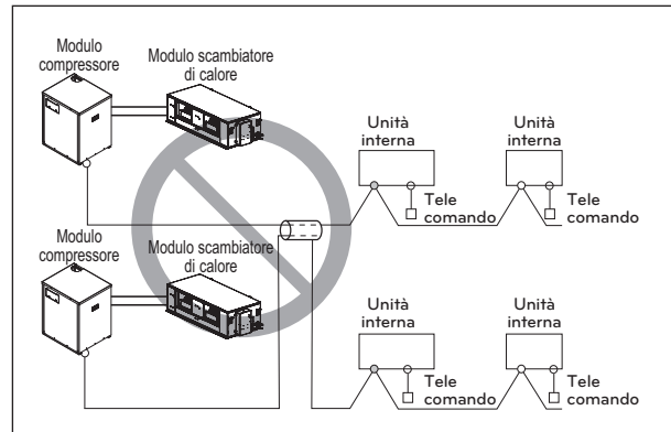
Cavo multiplo
