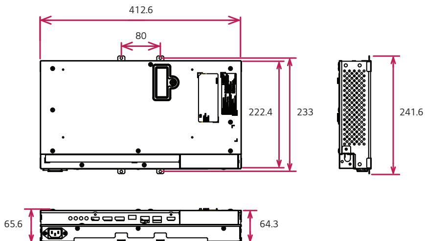
&lt;Signage Box&gt;
