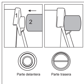
Figura 1. Instalación de los topes (no en todos los modelos)
