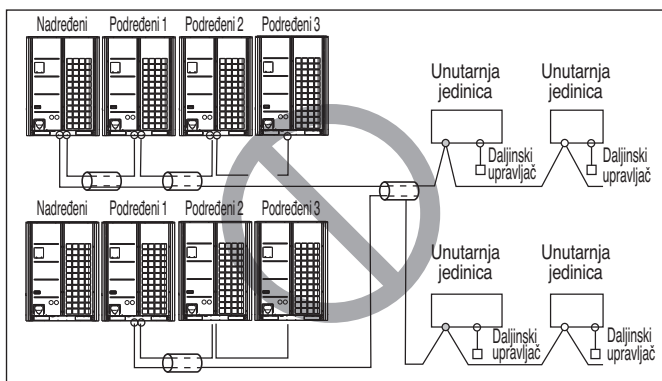
Višežilni kabel
