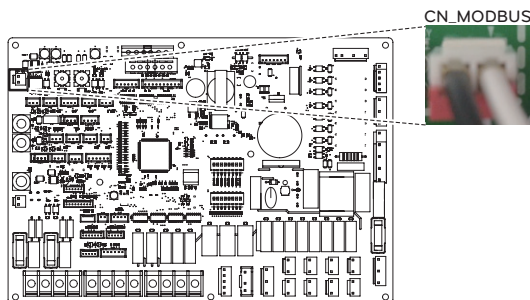
PCB interna
