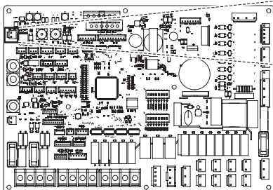
PCB interna
