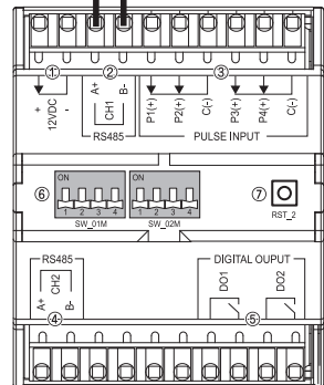
Interfaccia misuratore
