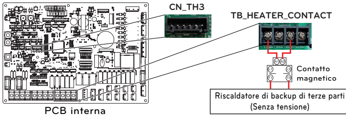
PCB interna
