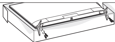
スタンド固定用ネジ (6本) M4 (長さ 20 mm)
