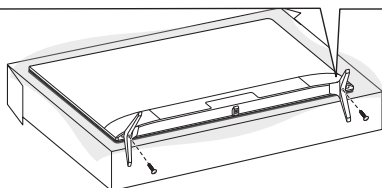
スタンド固定用ネジ (2本) M4 (長さ 16mm)
