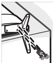
スタンド固定用ネジ (6本) M4 (長さ 20 mm)
