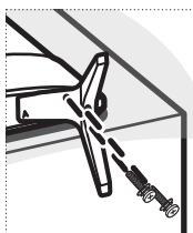
スタンド固定用ネジ (4本) M4 (長さ 20 mm)
