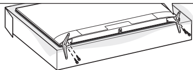
スタンド固定用ネジ (4本) M4 (長さ 20 mm)
