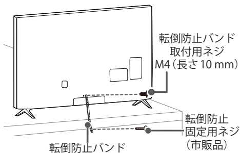
本体背面図
