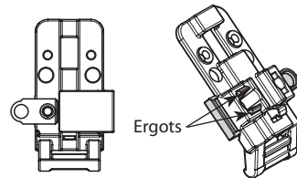
Assemblage de la charnière inférieure → b
