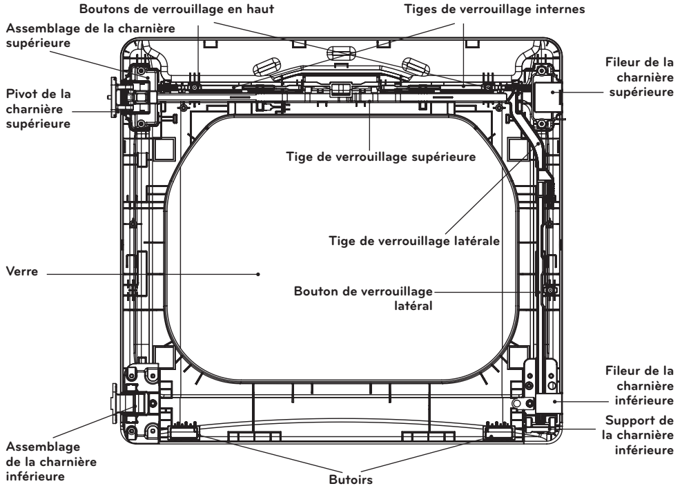
Structure interne de la porte (avant l'inversion, charnières à droite)
