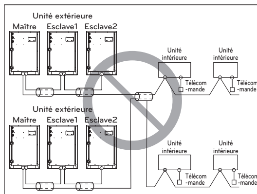
Câble multipolaire
