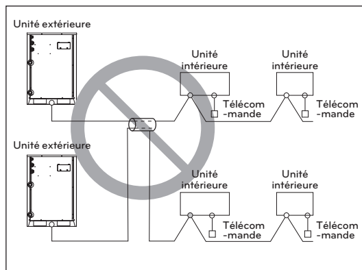
Câble multipolaire
