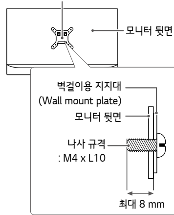
벽걸이용 지지대(Wall mount plate)
