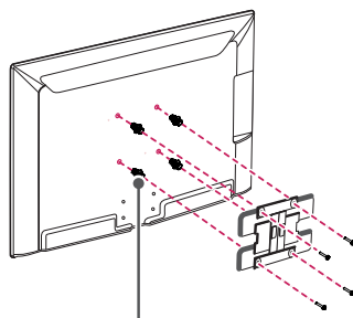
壁掛墊圈 (適用於 LA9700 系列)
