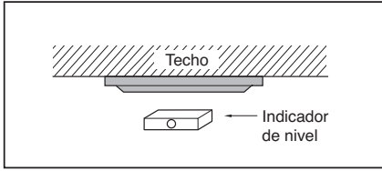
Chasis TQ/TR
