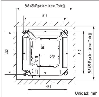
Chasis TQ/TR
