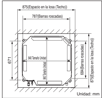
Chasis TM/TN/TP
