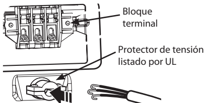
Cable eléctrico de cuatro hilos listado por UL
