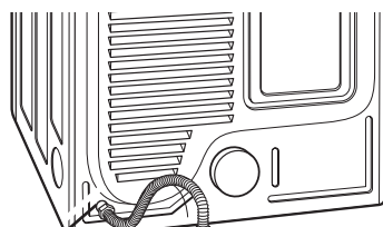
Conexión de gas \frac{3}{8} " NPT Conector flexible de acero inoxidable certificado por AGA/CSA Tapón de tubería de \frac{1}{8} " NPT Válvula de corte de suministro de gas
