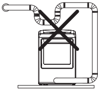
Tubería demasiado larga o con demasiados codos
