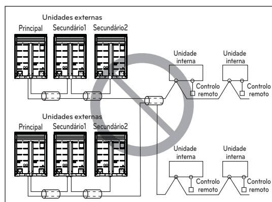
Cabo multi-núcleo
