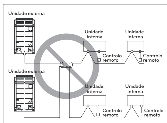
Cabo multi-núcleo
