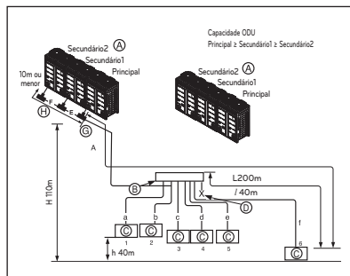
(Tabela 2) O diâmetro do tubo de refrigerante da unidade de exterior até a primeira ramificação (A)
