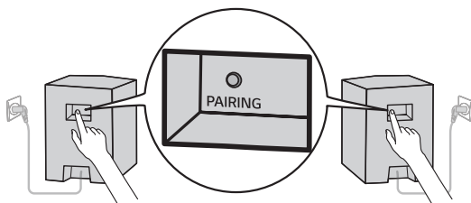
Conectarea manuală a difuzoarelor wireless spate
