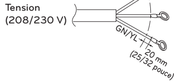
Cordon d'alimentation
