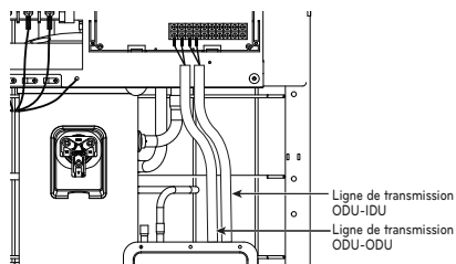
Raccordement du câble de communication
