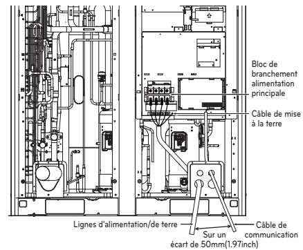
Façade avant 2
