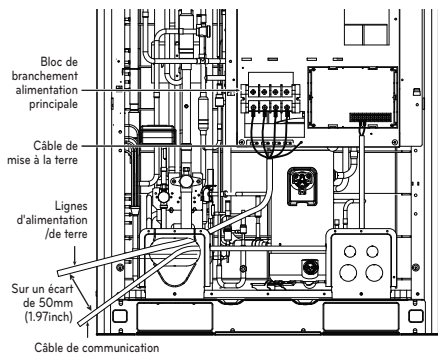
Façade avant 1
