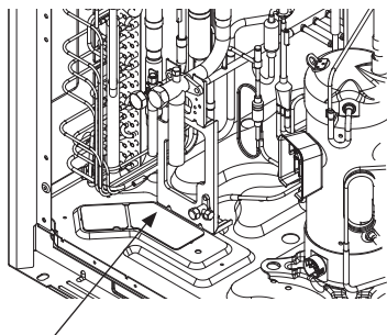
Zone d'extraction pour les raccords latéraux et les raccords de fond du tuyau de gaz/liquide
