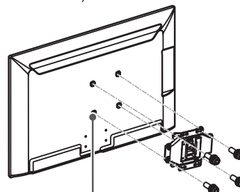
Inneres Distanzstück für Wandhalterung (Abhängig vom Modell)
