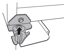
下部铰链
