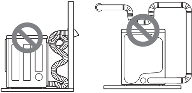
Conducto demasiado largo o muy torcido Tubería demasiado larga o con demasiados codos
