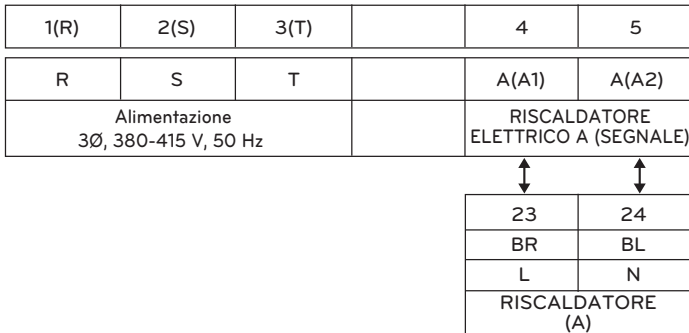
Morsetteria 3 (nell'unità)
