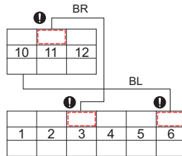
Morsettiera 3 (Unità interna)
