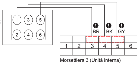
Morsettiera 3 (Unità interna)
