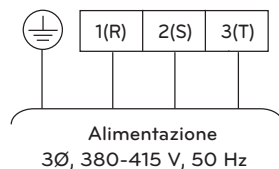
Morsettiera 2 (in riscaldatore di riserva 3Ø)
