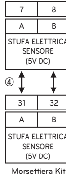
Morsettiera 1 (Nel Riscaldatore integrativo)
