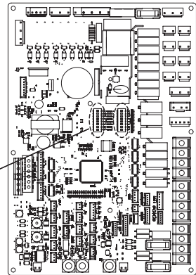
(Unità interna per R32 Hydrosplit, Unità Per Monobloc 4 serie)
