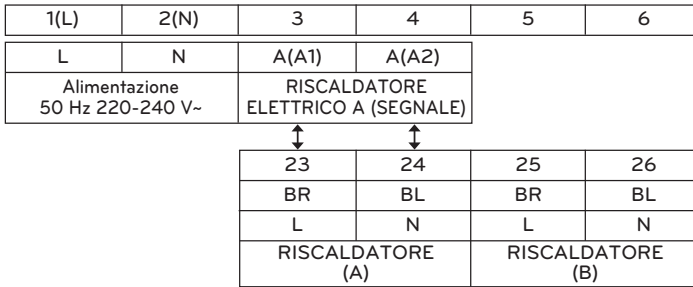
Morsetteria 3 (nell'unità)
