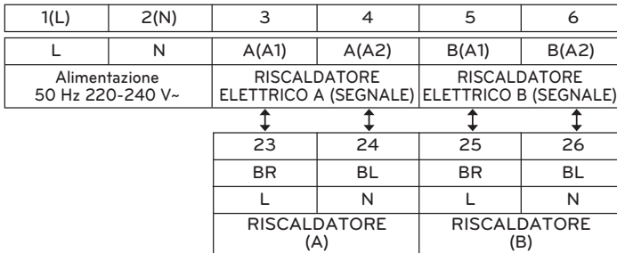
Morsetteria 3 (nell'unità)
