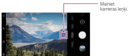
Aizmugures kamera
