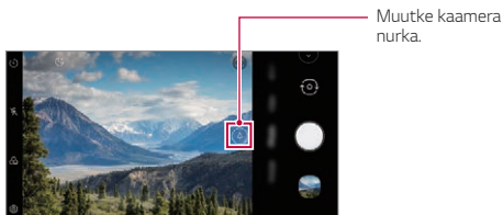
Tagakülje kaamera
