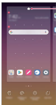
Výchozí obrazovka
