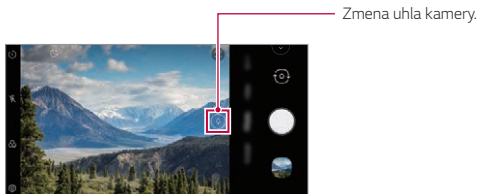
Zadný fotoaparát
