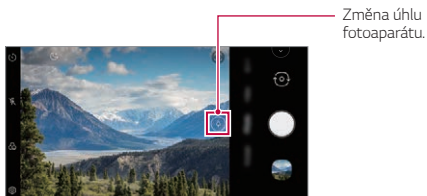
Zadní fotoaparát
