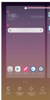
Noklusējuma ekrāns
